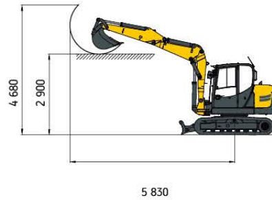
Fig. 3: Hauteur de chargement
