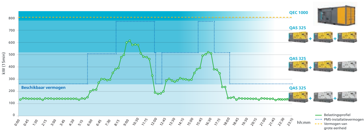
Let op: deze gegevens zijn nagebootst. Ze zijn gebaseerd op een kenmerkend industrieel belastingsschema.
