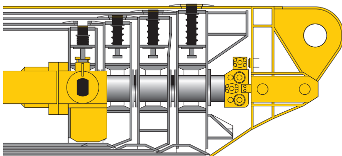
perfil de pluma ovalado
