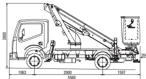
142TLE sur porteur MAXITY CABSTAR
