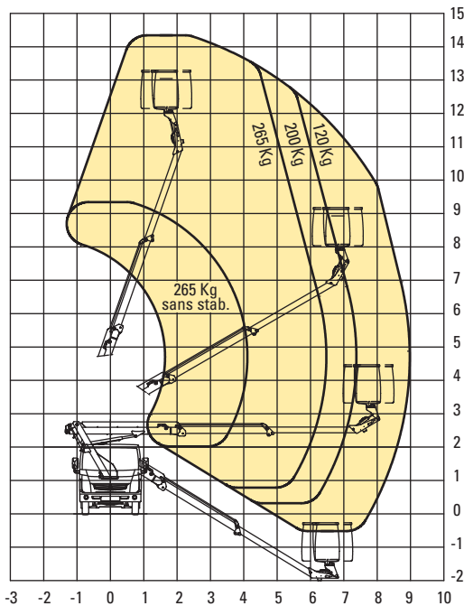
Courbe de travail - Working curve 142TLE
