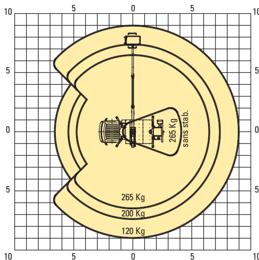
142TLE sur porteur MAXITY CABSTAR
