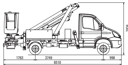
142TLE sur porteur IVECO
